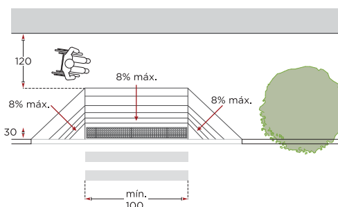
Rampa con lados alabeados
